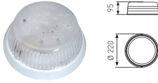
DEKORATİF TAVAN ARMATÜRÜ (YILDIZ)
