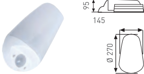
SENSÖRLÜ DUVAR APLİK
