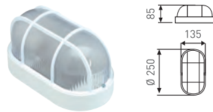
KAFESLİ ARMATÜR
